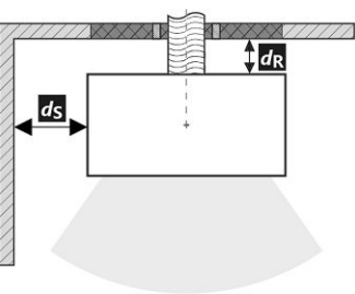
Hinterer Rauchrohranschluss
