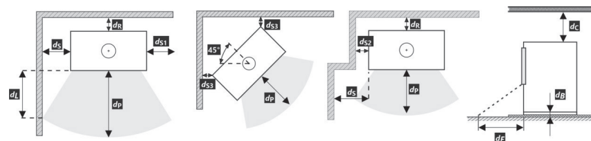
Fig. 2 Distanza di materiali infiammabili
