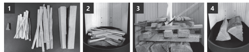
Fig. 4 Preparazione del combustibile per l'accensione iniziale
