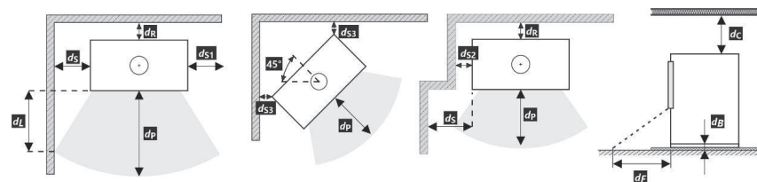
Abb. 2 Abstand zu brennbaren Materialien
