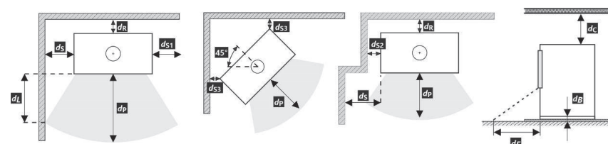
Fig. 2 Distance de sécurité du produit aux matériaux
